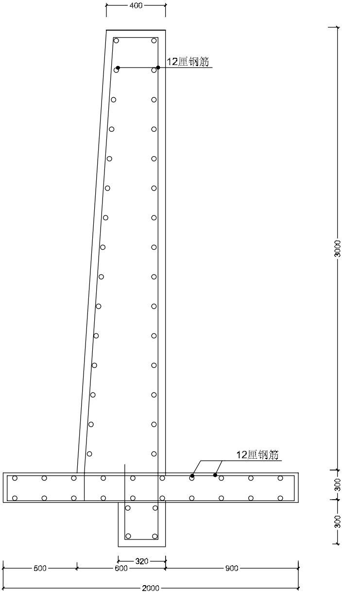
挡土墙示意图
